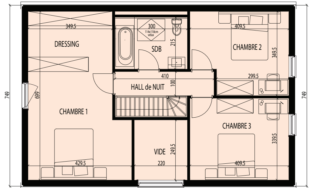
ETAGE - 85m 2
