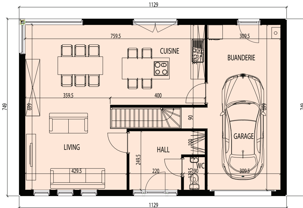
REZ-DE-CHAUSSEE - 85m 2
