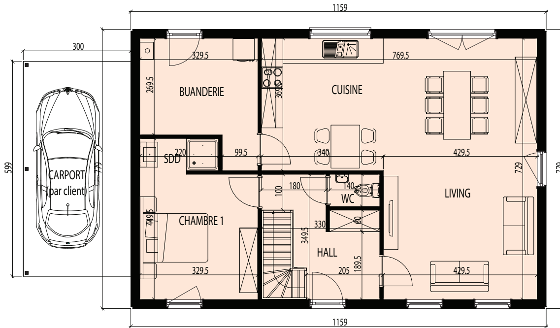
REZ-DE-CHAUSSEE - 90m 2
